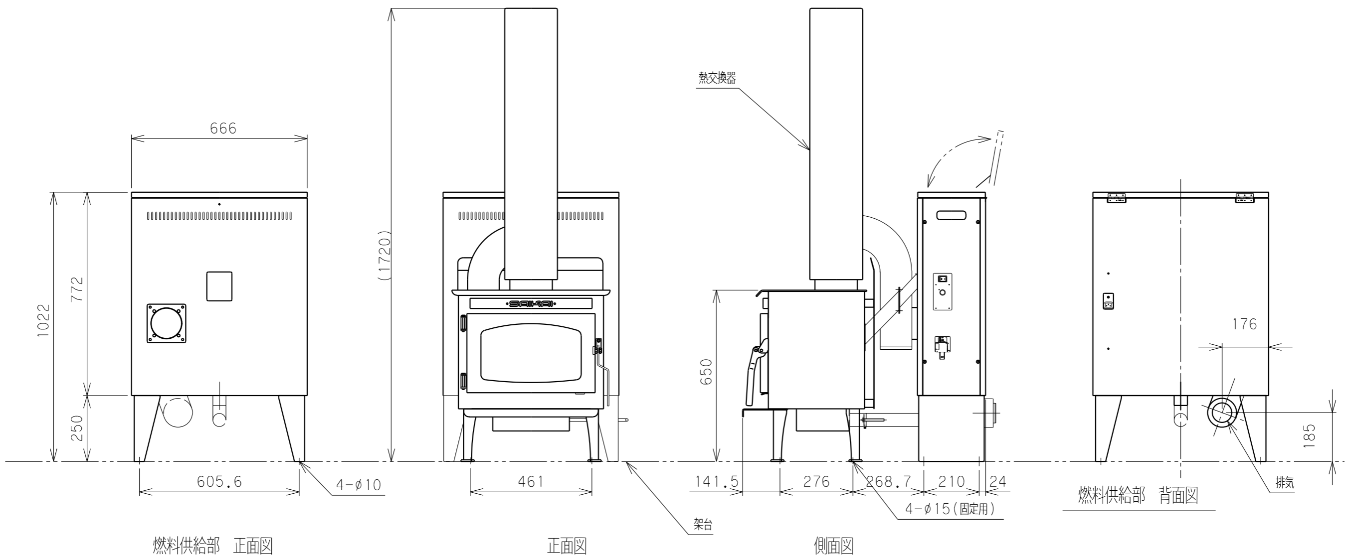
SAIKAI DK 外觀寸法図
